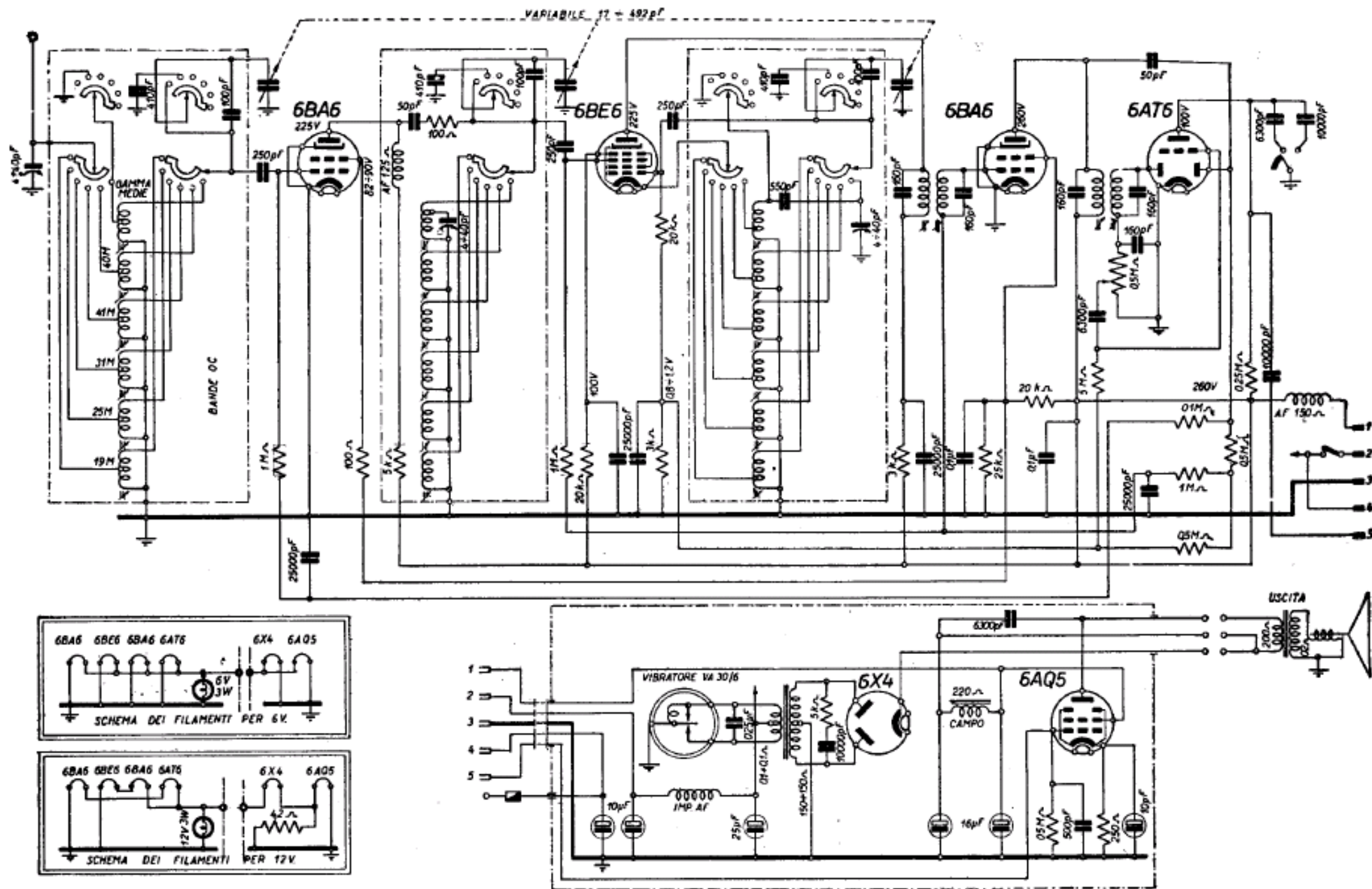
IRI « AUTOVOX » - Mod. RA7 - Gamma medie e cinque bande onde corte. Gruppo AF GS 7, gruppo alimentazione GA 7, altoparlante AP 12, antenna AS 1. Media frequenza a 455 kc.
